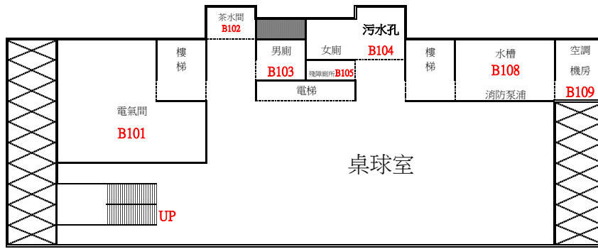
地下室平面圖
