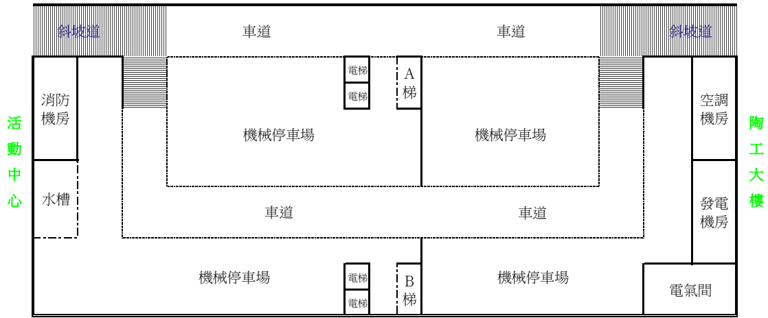
地下室平面圖
