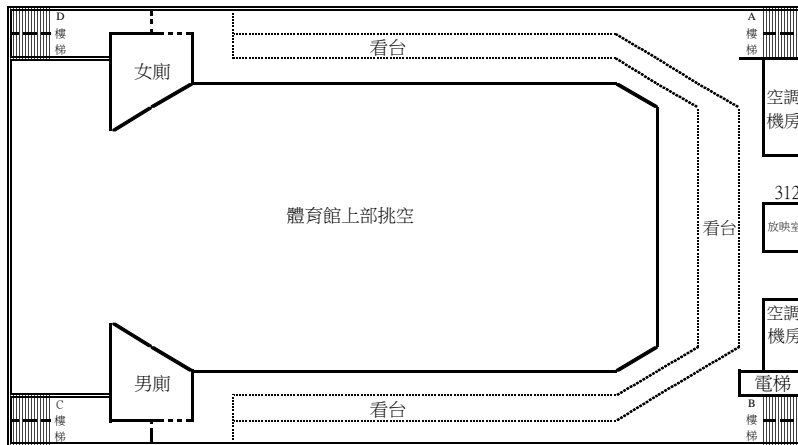
二樓平面圖
