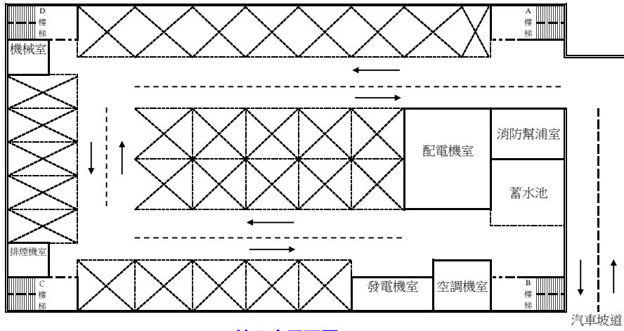
地下室平面圖
