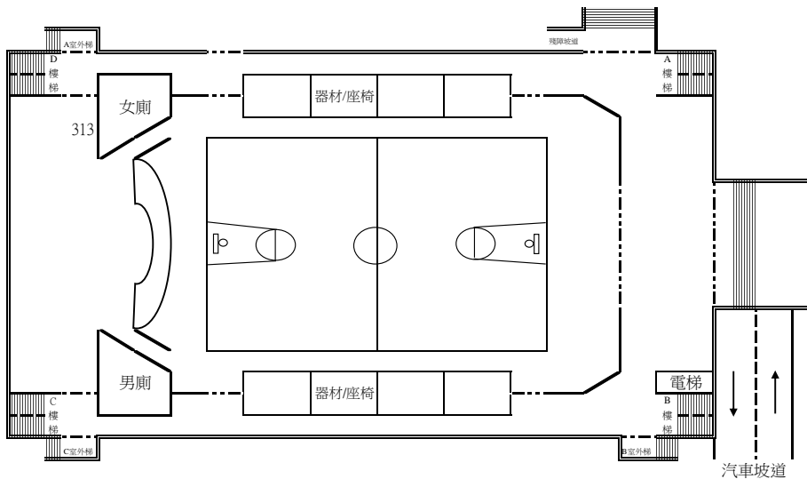
一樓平面圖
