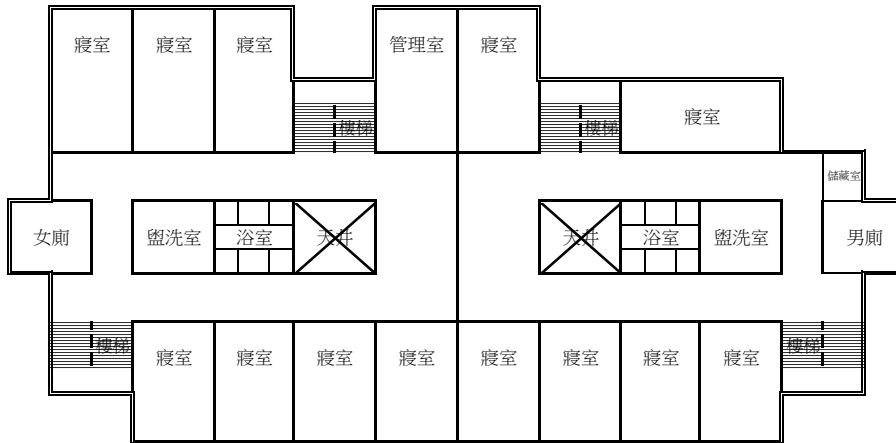
四樓平面圖
