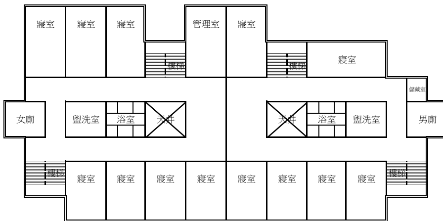
五樓平面圖
