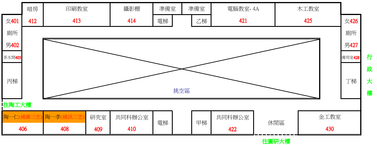
四樓平面圖
