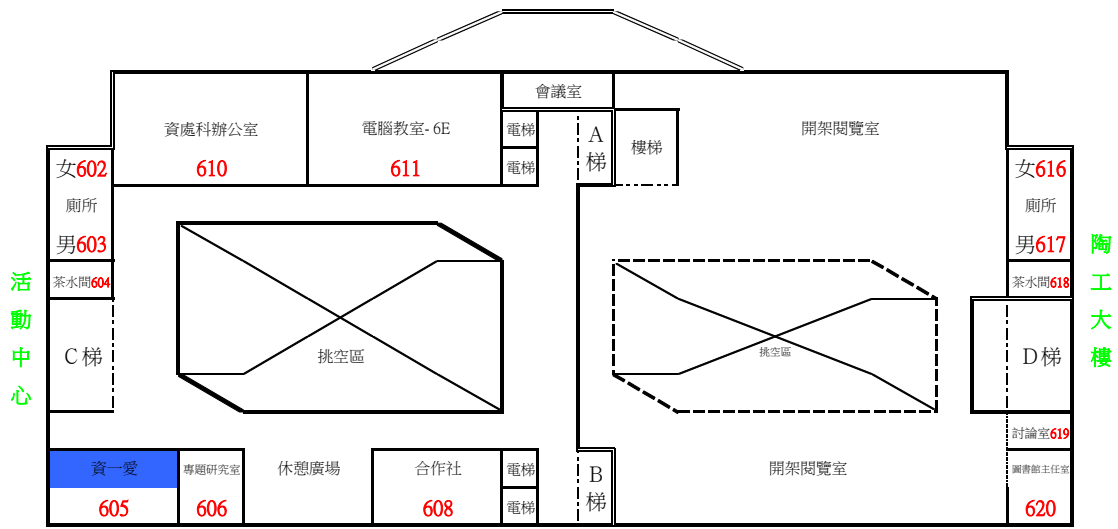
六樓平面圖
